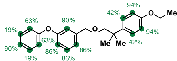
11. Etofenprox
