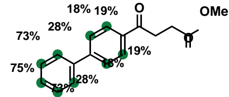
20. Fenbufen
