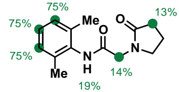
3. Nefiracetam
