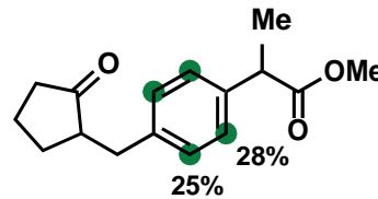
13. Ketoprofen
