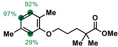
1. Gemfibrozil
