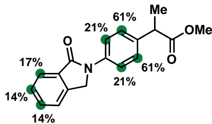
21. Indoprofen
