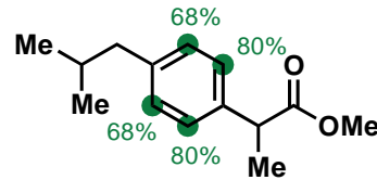
2. Ibuprofen
