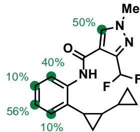
7. Sedaxane
