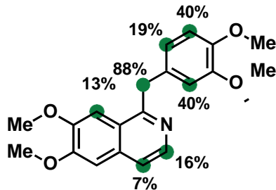
18. Papaverine
