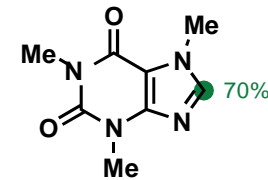
6. Caffeine
