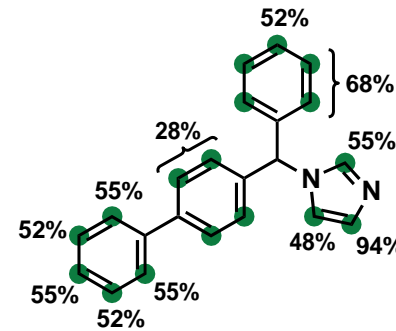
17. Bifonazole
