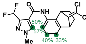
8. Benzovindiflupyr
