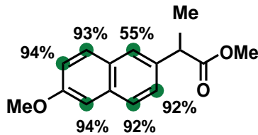
15. Naproxen
