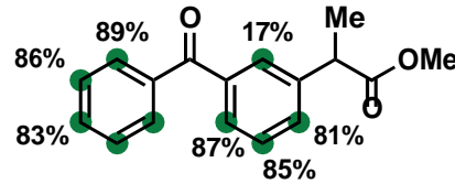
13. Ketoprofen
