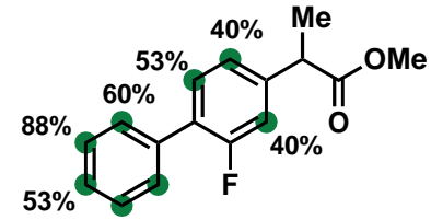
14. Flurbiprofen
