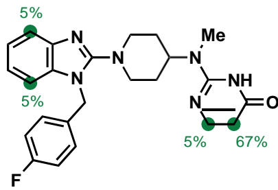
10. Mizolastine
