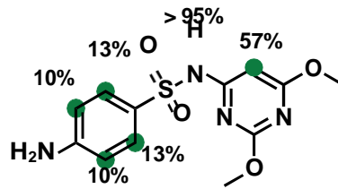
19. Sulfadimethoxine
